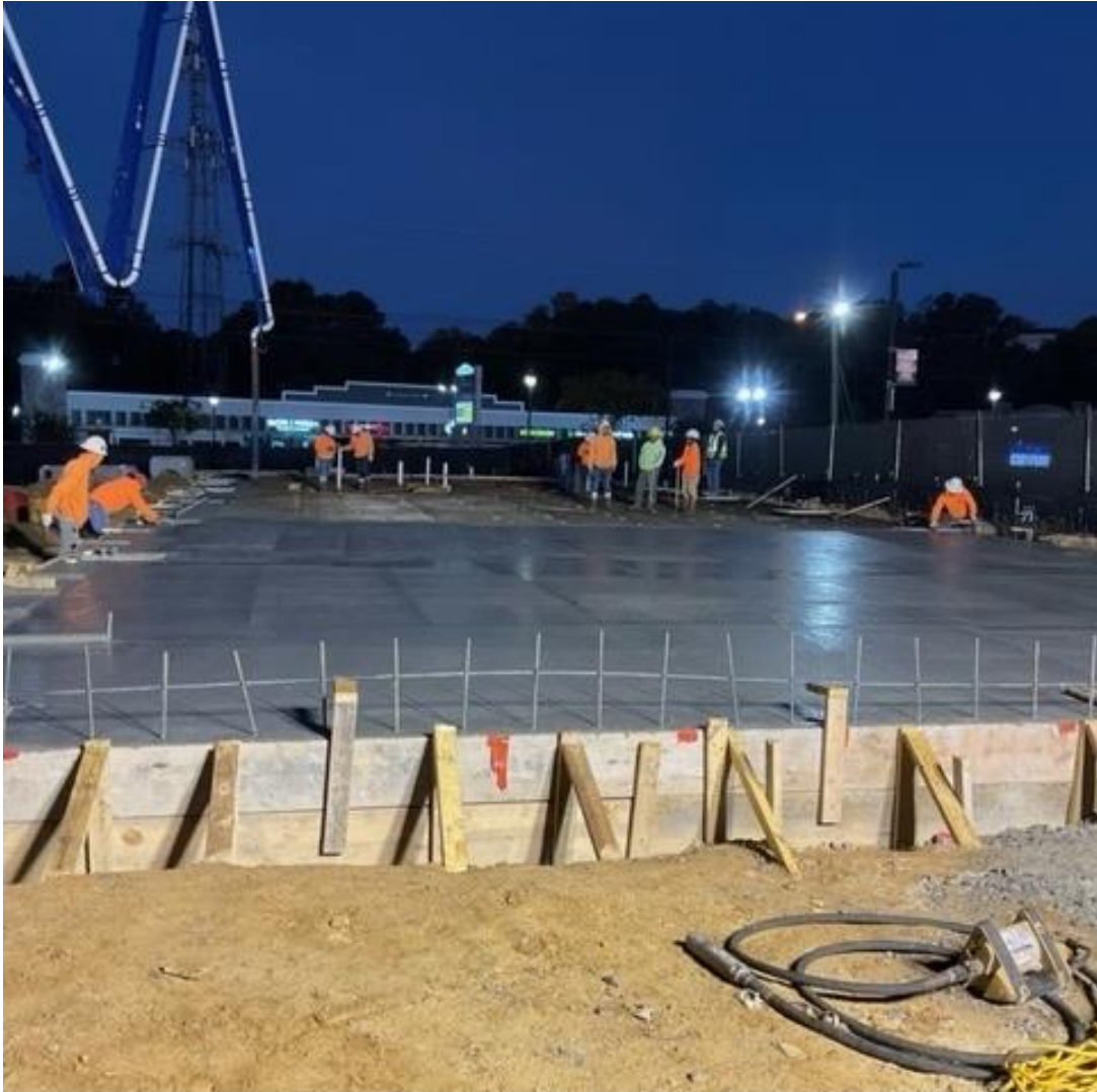
Pour SOG
